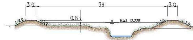
河川整備計画断面図（藤島川合流点から上流2.7km）
