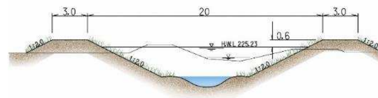
河川整備計画断面図（最上川合流点から上流8.5km）
