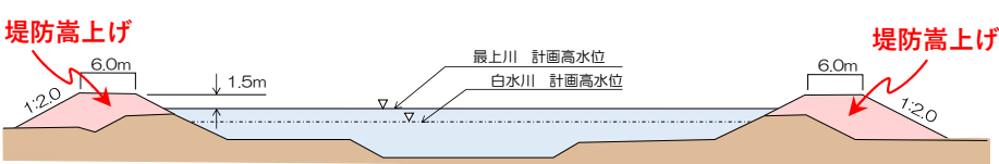
河川整備計画断面図
