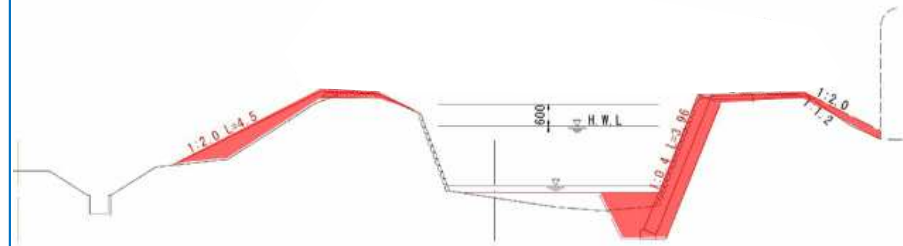
計画断面図
