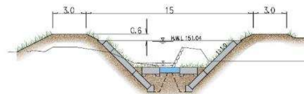
河川整備計画断面図 (国道13号橋から上流0.1km)
